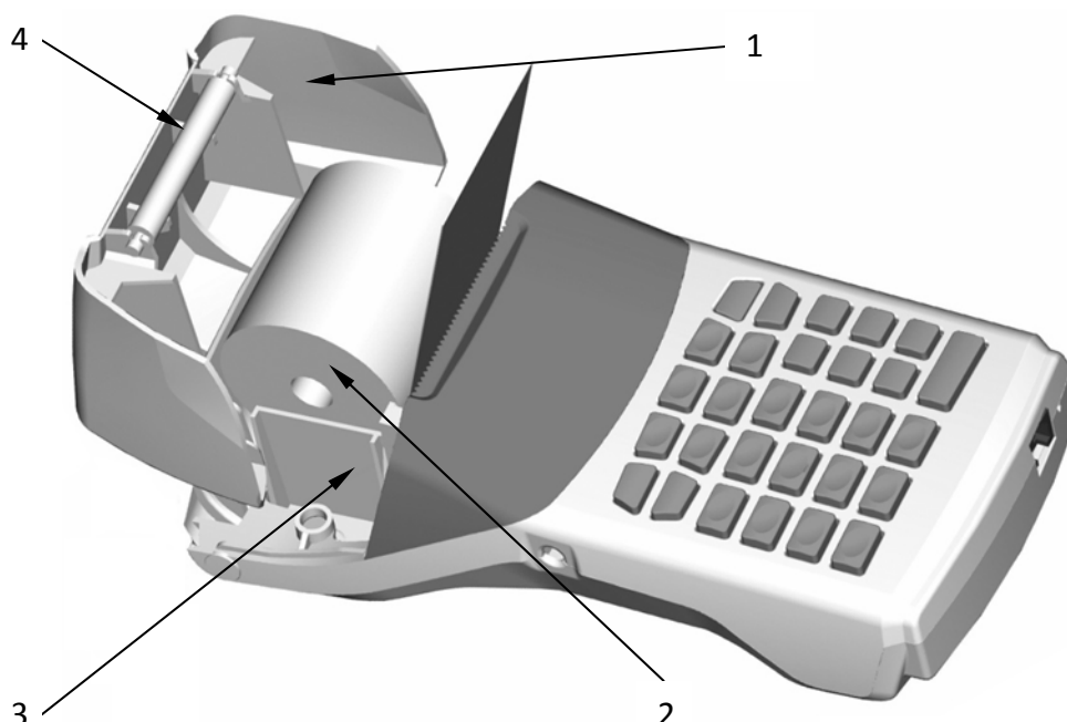
Рисунок 6 – Заправка бумаги в ЧПМ «ОРИОН-105».
