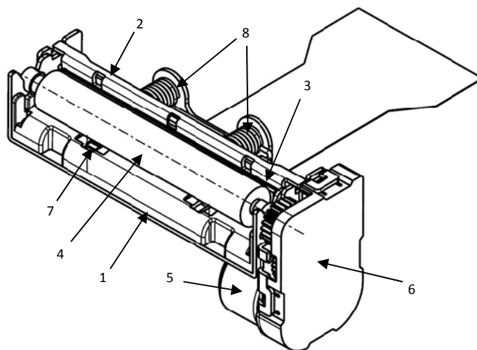
Рисунок 7 – Внешний вид ТПМ ЧПМ «ОРИОН-105».
