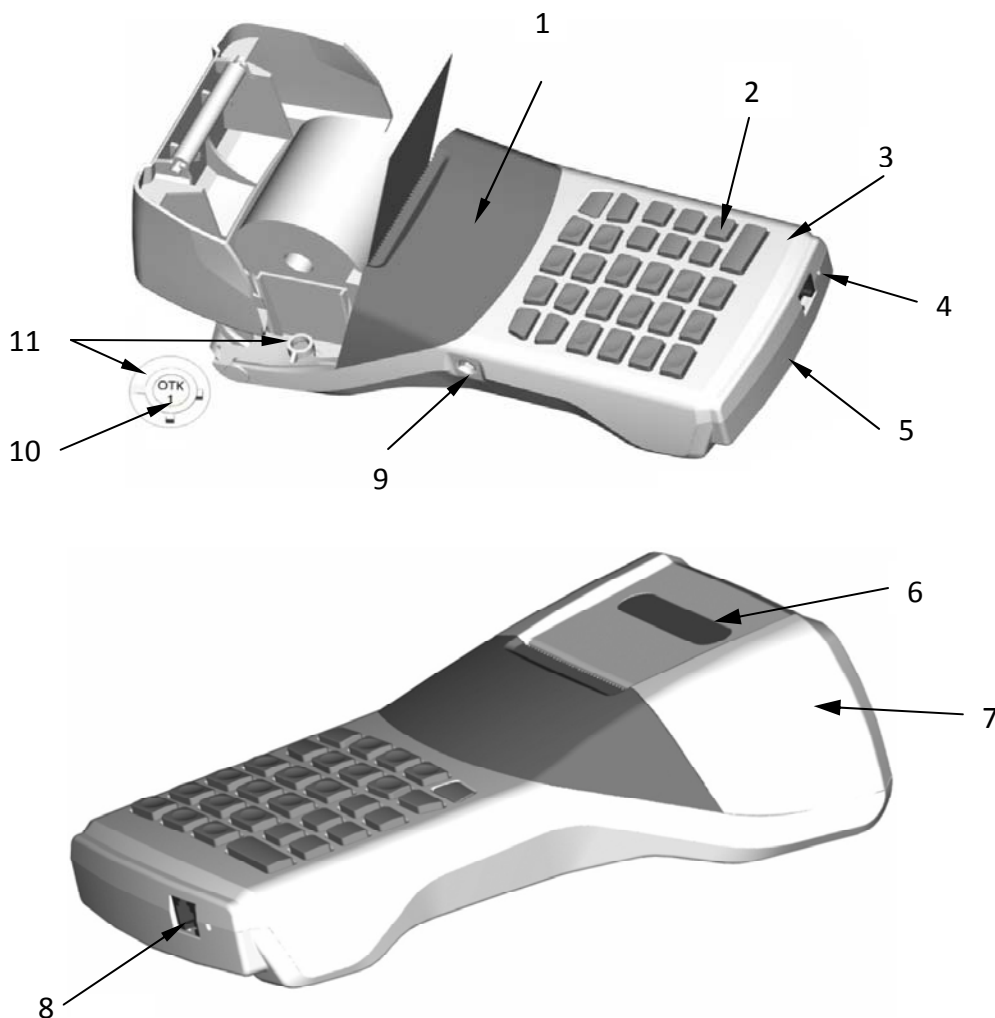
Рисунок 1 – Внешний вид ЧПМ «ОРИОН-105».
