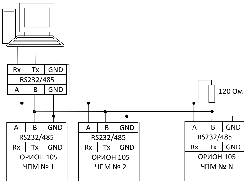
Рисунок 9 – Объединение в сеть ЧПМ «ОРИОН-105».
