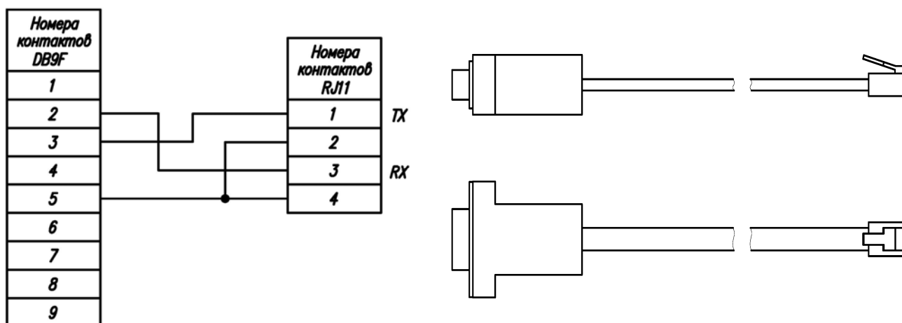
Рисунок 9 – Схема переходника DB9M – RJ11.
